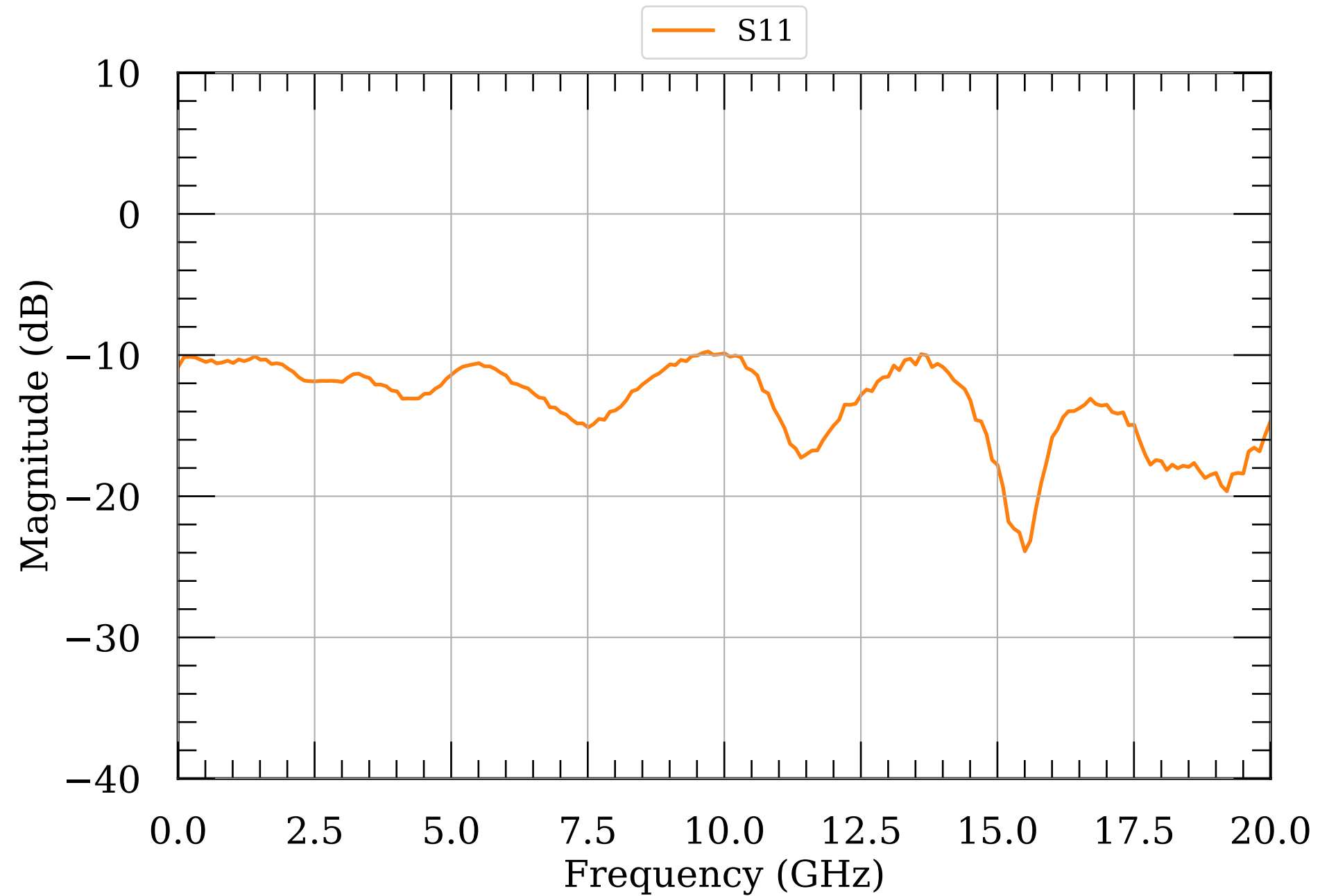
LNA S-params module018v2
